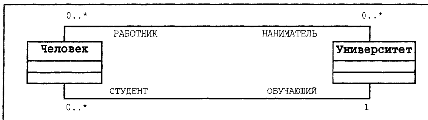
Рис. 10.9. Ассоциации с указанными кратностями ролей
