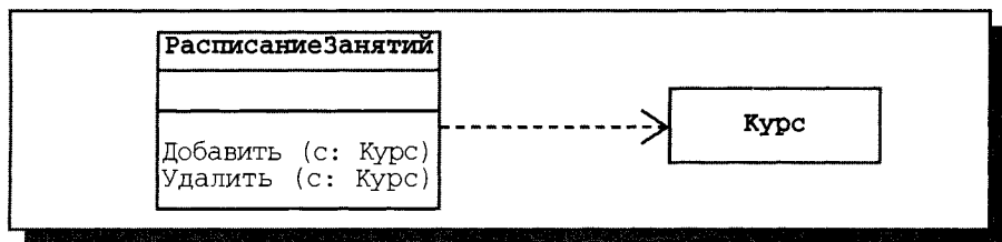
Рис. 10.4. Диаграмма классов со связью-зависимостью
