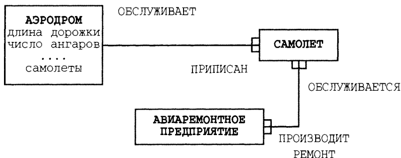
(б) Аналог ER-диаграммы после приведения к первой нормальной форме
