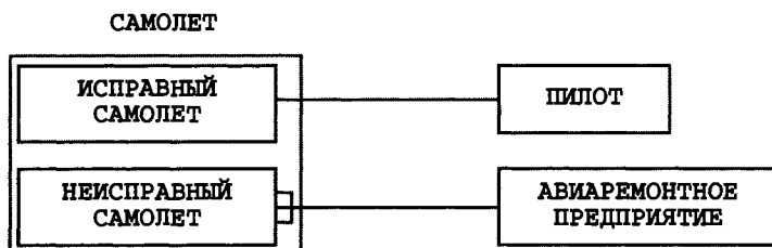
(б) Аналог без взаимно исключающих связей, но с подтипами
