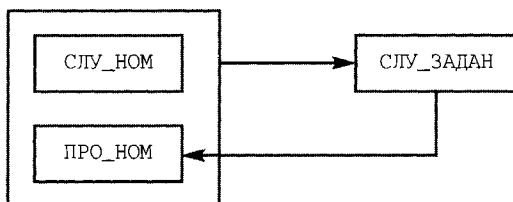
Диаграмма FD отношения СЛУЖ_ПРО_ЗАДАН (новый вариант)
