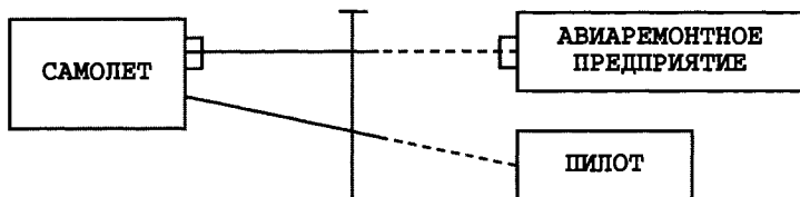
(а) ER-диаграмма со взаимно исключающими связями
