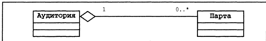
Рис. 10.10. Пример агрегатной ассоциации
