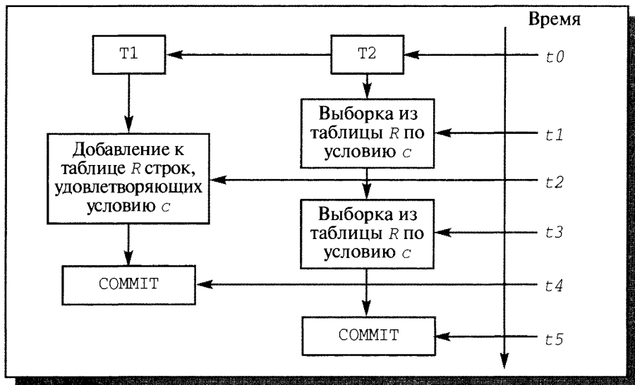
Рис. 18.6. Феномен фантомов
