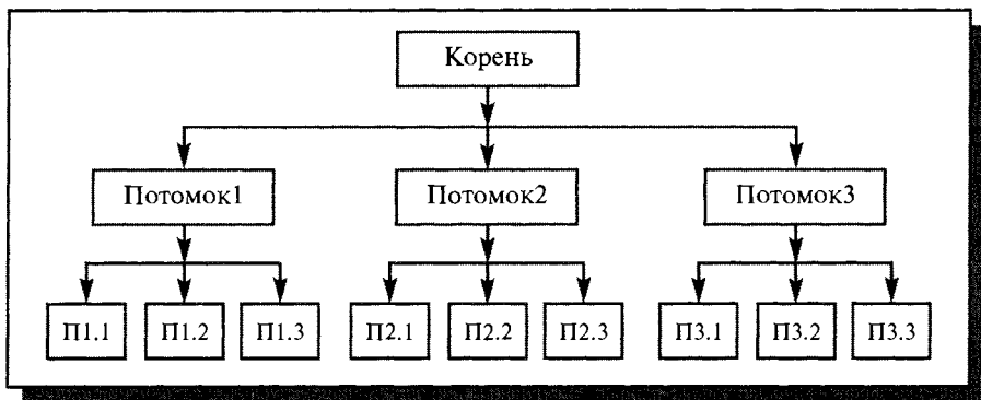
Рис. 16.5. Пример дерева
