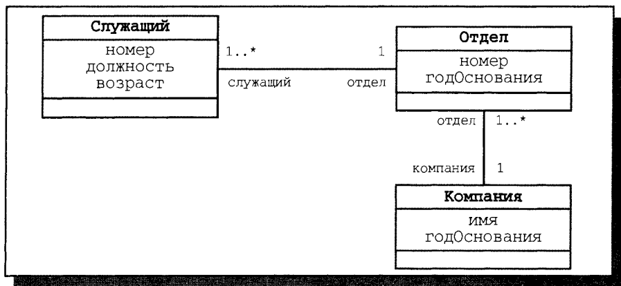
Рис. 10.14. Диаграмма классов, используемая для примеров на языке OCL
