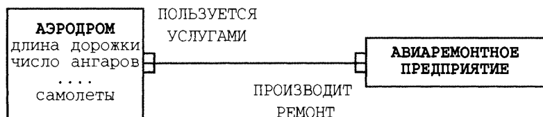
(а) ER-диаграмма, не находящаяся в первой нормальной форме
