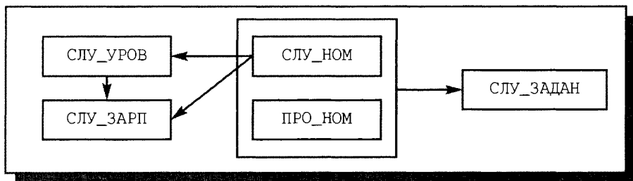
Рис. 7.1. Диаграмма множества FD отношения СЛУЖАЩИЕ_ПРОЕКТЫ_ЗАДАНИЯ
